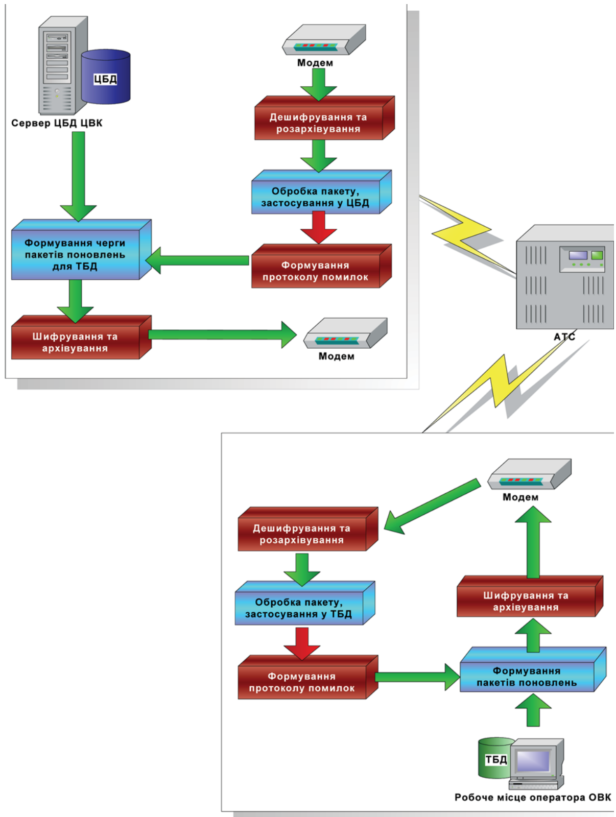
Рис. 2. Схема обміну інформацією між центральною базою даних Центральної виборчої комісії (ЦБД ЦВК) та територіальними базами даних (ТБД ОВК) окружних виборчих комісій
