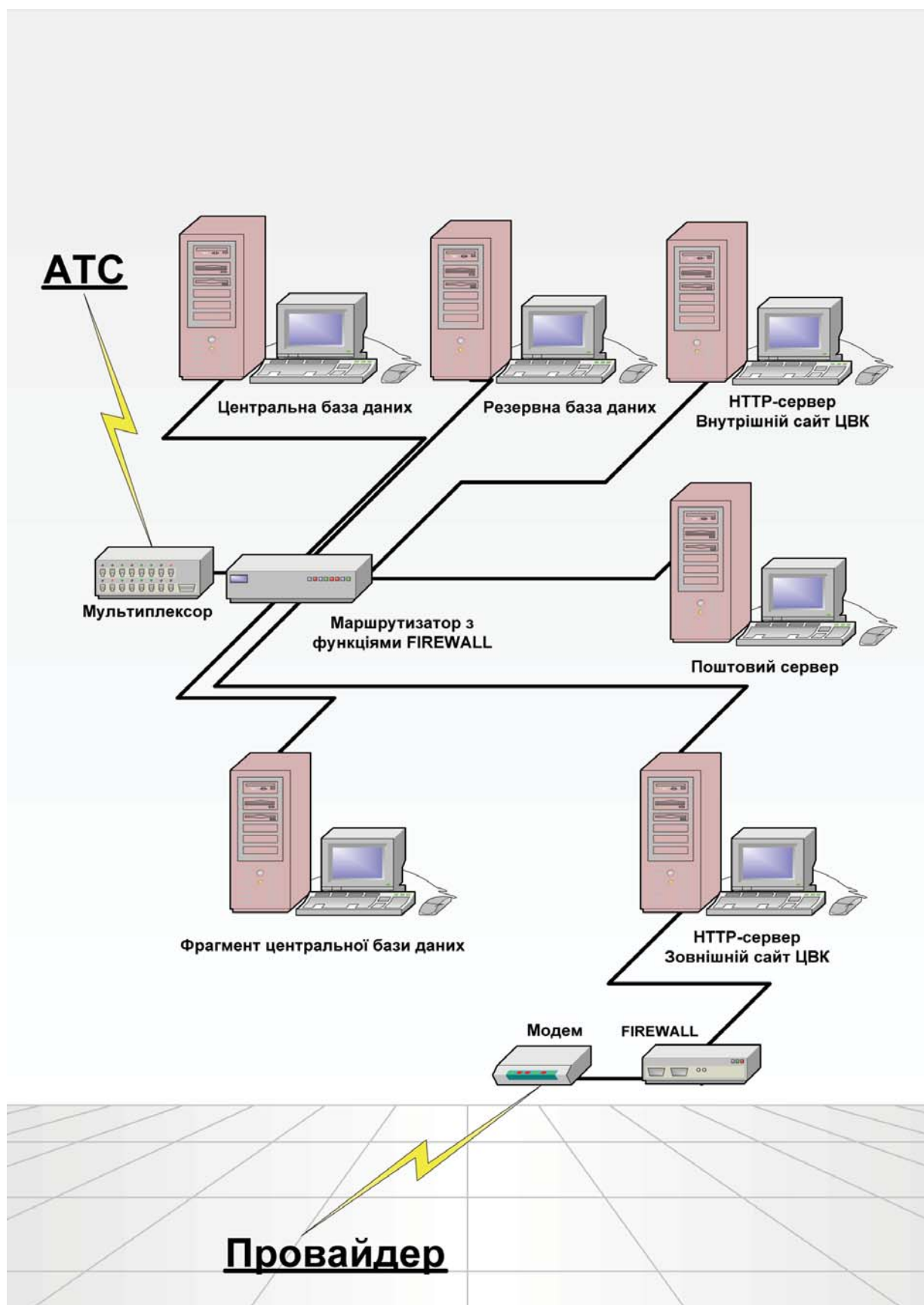
Рис. 8. Основні технічні засоби інформатизації виборчого процесу Центральної виборчої комісії
