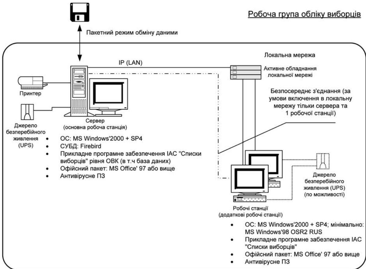
Рис. 6. Архітектура програмно-технічного комплексу системи на регіональному та місцевому рівнях
